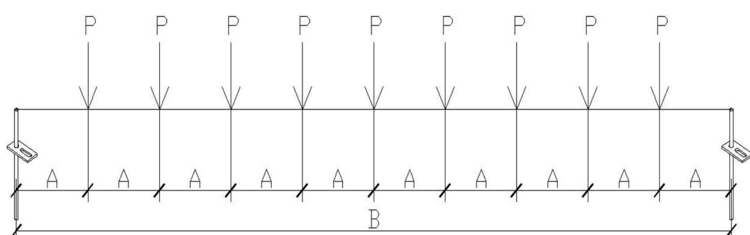
Diagramma delle tensioni. Diagramma di carico a rottura
